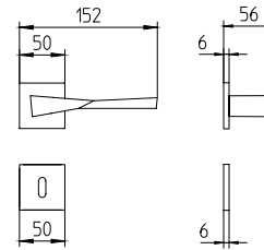
1691 maniglia per porta con rosetta door handle on rose
