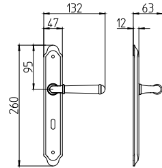
1340 con piastra on backplate
