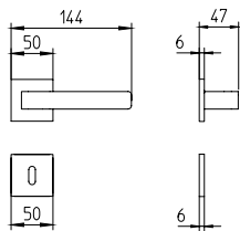
1681 maniglia per porta con rosetta door handle on rose
