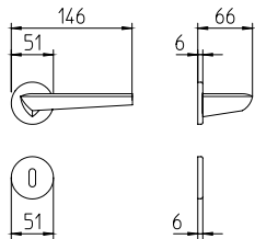
1081 maniglia per porta con rosetta door handle on rose
