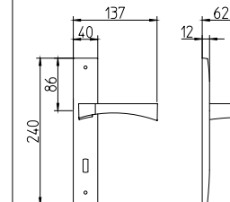
1170 con piastra on backplate
