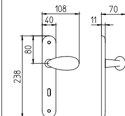
1090 con piastra on backplate
