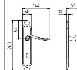
1020 con piastra on backplate
