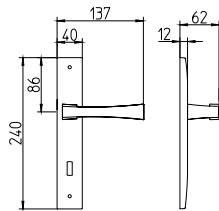
1160 con piastra on backplate
