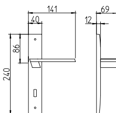
1370 con piastra on backplate
