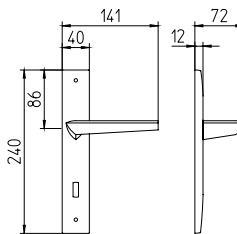
1080 con piastra on backplate
