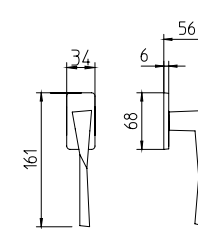
1692/DK martellina dk drehkipp system
