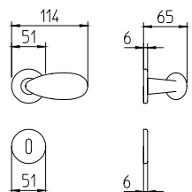
1091 maniglia per porta con rosetta door handle on rose
