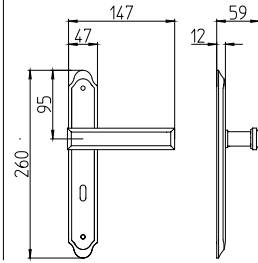
1740 con piastra on backplate
