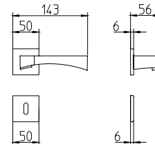
1171 maniglia per porta con rosetta door handle on rose
