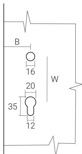
Maniglia con bocchetta foro cilindro standard e slim Handle with standard or slim cylinder hole escutcheon
