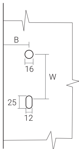
Maniglia con bocchetta foro chiave standard e slim Handle with standard or slim key hole escutcheon
